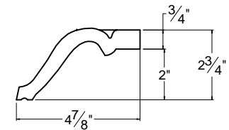
End Elevation
