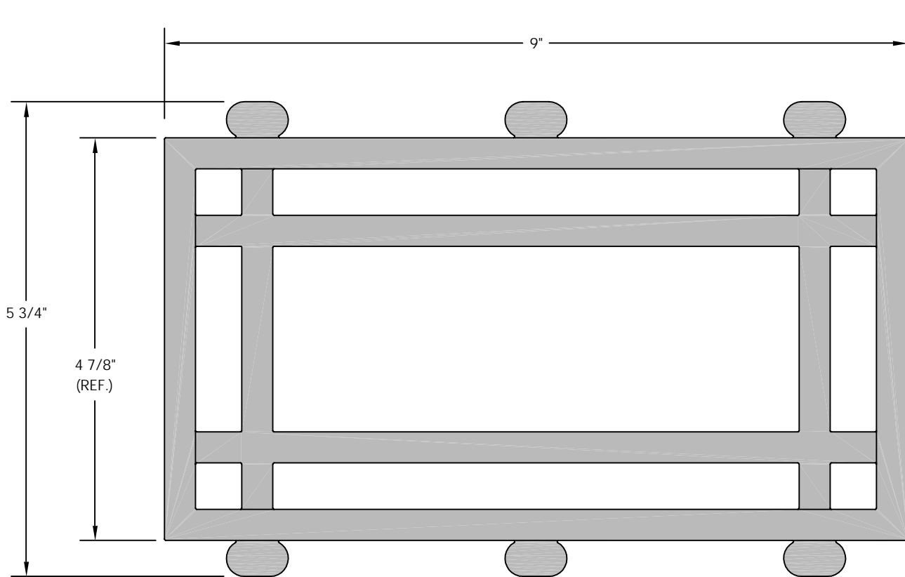
ELEVATION
