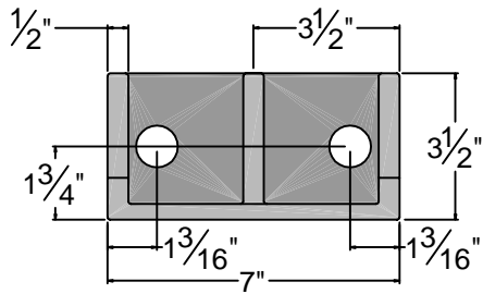
Bottom Elevation
