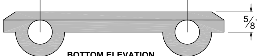
BOTTOM ELEVATION
